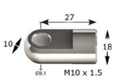
#62.127 Eye M10x27
